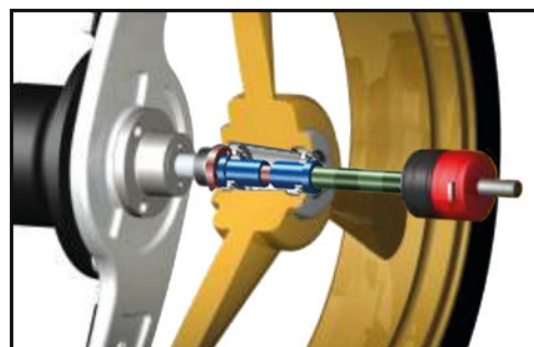
Albero con bussole di centraggio
