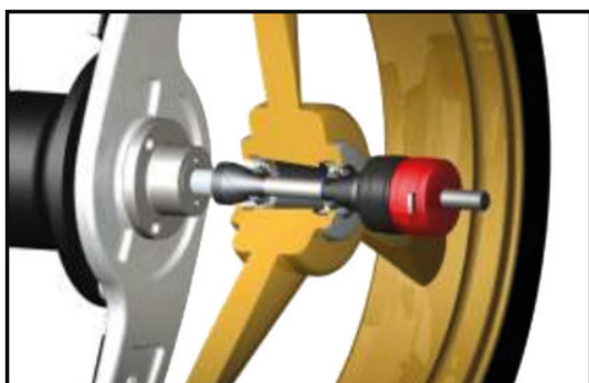
Albero con coni di centraggio
